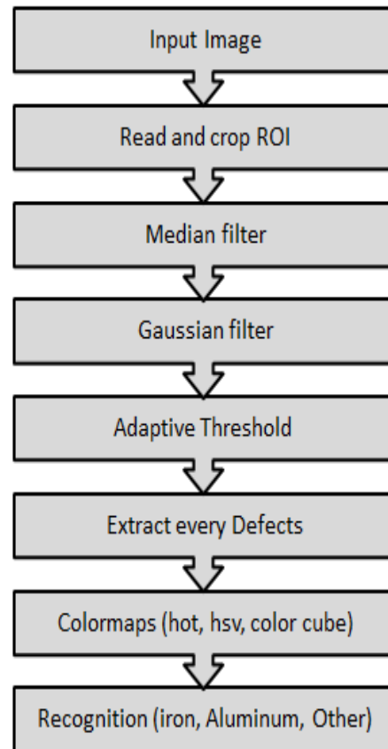
شکل ۳- ساختار سیستم ICAS
